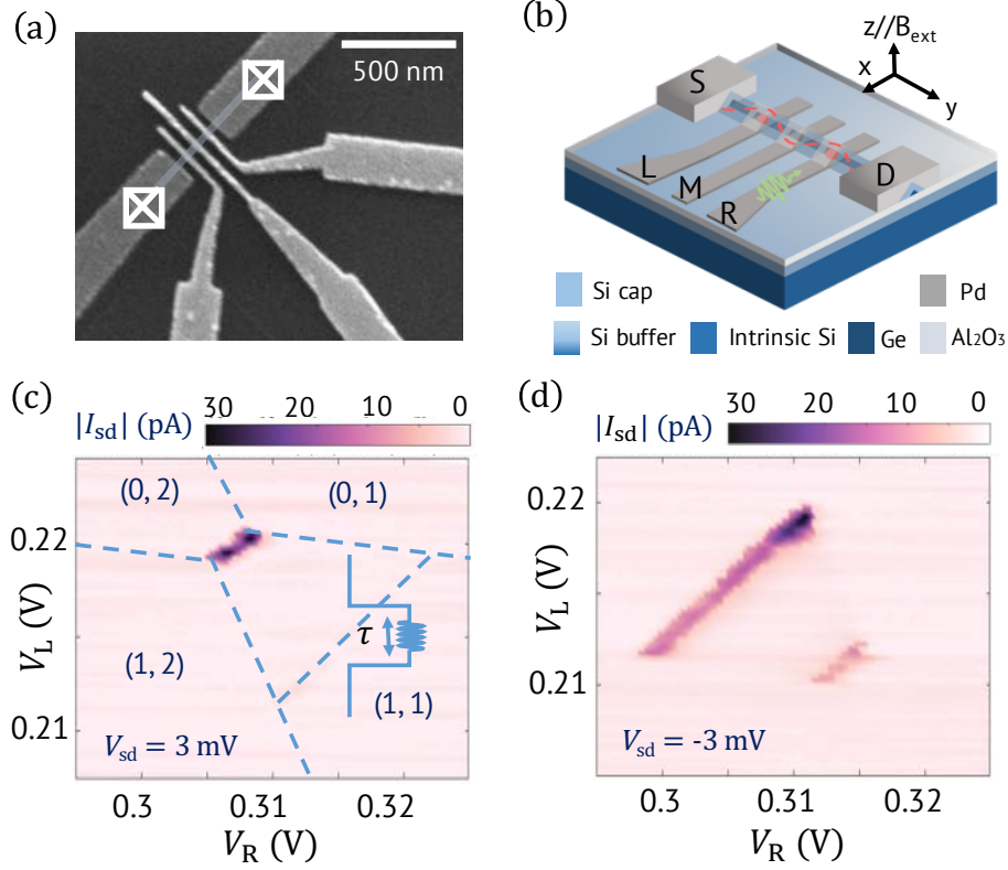
图 5.3 (a) 锗硅纳米线双量子点的 SEM 结构实物图和纳米线方向的切面示意图。SEM 图中白色盒子代表欧姆接触。(b) 双量子点结构的示意图，通过外加在电极 L, M 和 R 上的直流电压对纳米线中的势垒进行调控，最终在电极 L 和 R 下方附近形成双量子点，电极 M 可以调制两个量子点之间的耦合作用大小。直流电压 R 电极除了添加直流电压外，在进行比特控制时，微波和脉冲信号也从该电极进入器件。门电极与源漏电极之间由氧化铝绝缘层进行隔离。实验中外加磁场垂直于基片。(c) 扫描电极 L 和 R 得到的“偏压三角形”电荷稳态图，从相图中可以得知，量子点形成位置基本处于 L 和 R 金属电极的下方。方波信号代表比特操作时的方向。(d) 负偏压下的“偏压三角形”电荷稳态图，在失谐量为零处仍然存在较大的电流信号。
